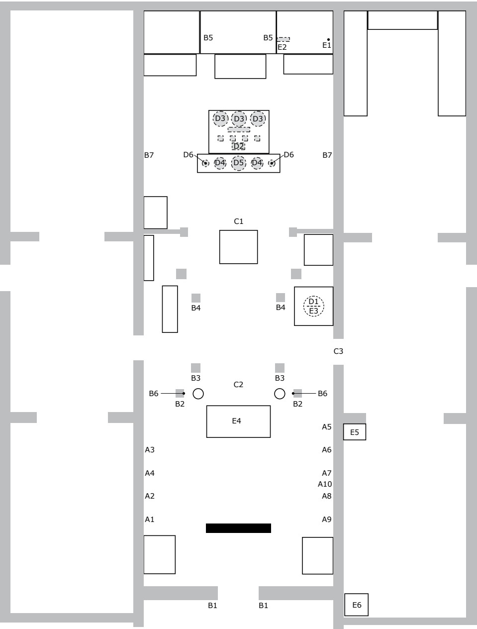
洪聖古廟器物位置圖
